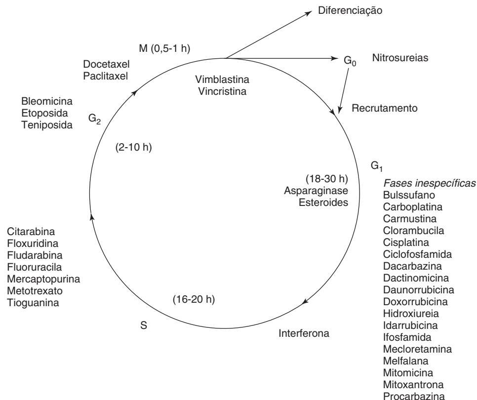
FIGURA 42-1 Locais de atividade antineoplásica no ciclo celular. G 0 , fase de repouso; G 1 , período antes da síntese do DNA, durante o qual são sintetizadas as enzimas necessárias para a síntese do DNA; G 2 , período de síntese do RNA e de proteínas especializadas, assim como a produção do aparelho do fuso mitótico; M, mitose, S, síntese do DNA, durante a qual o DNA é replicado.
