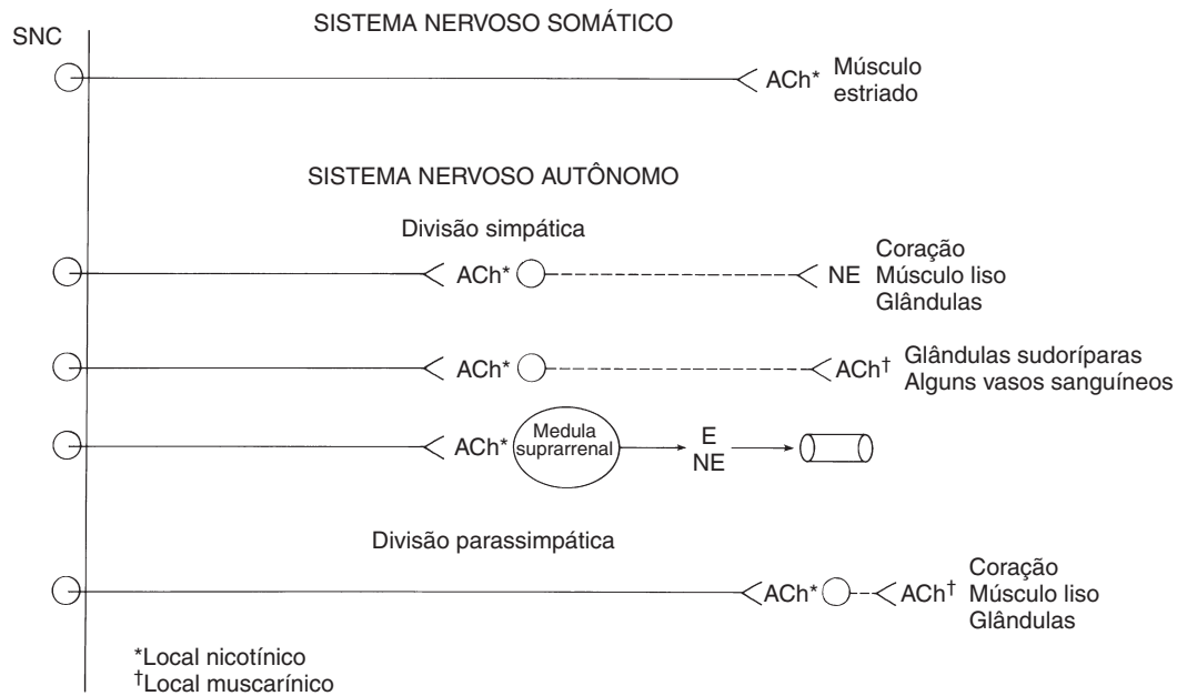
FIGURA 5-1 Organização funcional do sistema nervoso somático e do sistema nervoso autônomo, com as estruturas inervadas pelos diferentes neurônios e os mediadores químicos responsáveis pela transmissão nos vários locais. Linhas contínuas indicam neurônios somáticos motores ou autonômicos pré-ganglionares; linhas tracejadas indicam neurônios autonômicos pós-ganglionares. ACh, acetilcolina; E, epinefrina; NE, norepinefrina.
