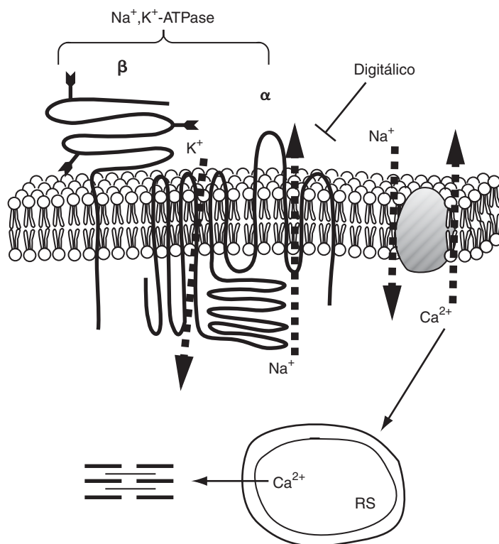
FIGURA 25-6 Papel da \text{Na}^+/\text{K}^+ -ATPase e da troca \text{Na}^+-\text{Ca}^{2+} na contratilidade e o mecanismo do efeito inotrópico positivo da digoxina. A digoxina liga-se à face extracelular e à região transmembrana da subunidade \beta da \text{Na}^+/\text{K}^+ -ATPase, inibindo o efluxo de \text{Na}^+ e o influxo de \text{K}^+ . A subunidade \alpha ( \alpha ) da \text{Na}^+/\text{K}^+ -ATPase também é ilustrada. O aumento da concentração intracelular de \text{Na}^+ causa redução da ligação do \text{Ca}^{2+} ao sistema de troca \text{Na}^+-\text{Ca}^{2+} e diminuição do efluxo de \text{Ca}^{2+} . A concentração intracelular de \text{Ca}^{2+} aumenta e mais \text{Ca}^{2+} é disponibilizado para os sítios de armazenamento intracelulares, notadamente o retículo sarcoplasmático (RS). Decorre daí maior liberação de \text{Ca}^{2+} para o aparelho contrátil e maior força de contração.
