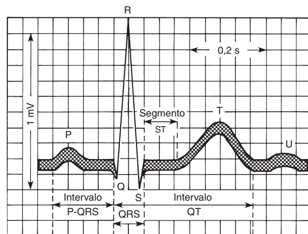
FIGURA 24-5 ECG normal. P, despolarização atrial; QRS, despolarização ventricular; T, repolarização ventricular. A onda U corresponde à repolarização interventricular. (De Milnor WR: The ECG. In Mountcastle VB, editor: Medical physiology , ed 14, St Louis, 1980, Mosby.)
