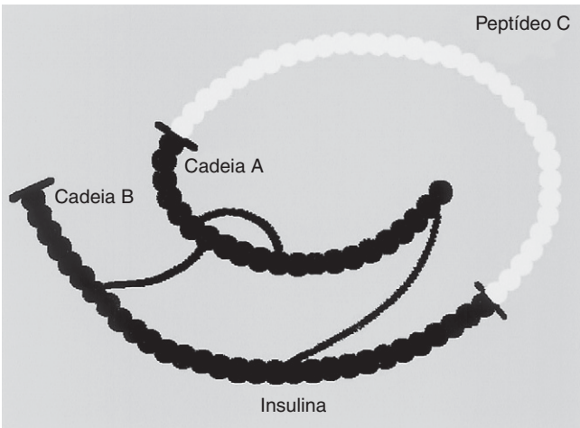
FIGURA 36-1 Estrutura da pró-insulina. Quando o peptídeo de conexão (C) é removido, forma-se a insulina. As cadeias A e B da insulina estão representadas em preto; o peptídeo C aparece em branco.
