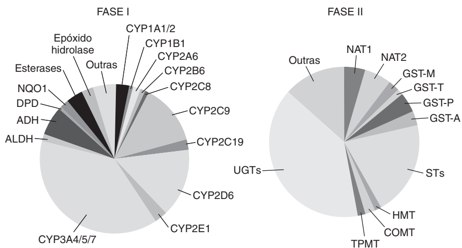
FIGURA 2-10 Principais enzimas envolvidas na biotransformação de fármacos. A porcentagem de contribuição de cada enzima no processo de biotransformação de fase I e de fase II de fármacos está representada pelo tamanho relativo de cada seção do gráfico correspondente. ADH , Álcool desidrogenase; ALDH , aldeído desidrogenase; CYP , citocromo P450; DPD , diidropirimidina desidrogenase; NQO1 , NAD(P)H:quinona óxido-redutase (ou DT diáforase); COMT , catecol-O-metil transferase; GST , glutathione S-transferase; HMT , histamina metiltransferase; NAT , N-acetiltransferase; STs , sulfotransferases; TPMT , tiopurina metiltransferase; UGTs , uridina difosfato glicuronosil-transferases. (Adaptado de Evans WE, Relling MV: Pharmacogenomics: translating functional genomics into rational therapeutics, Science 286:487-491, 1999.)
