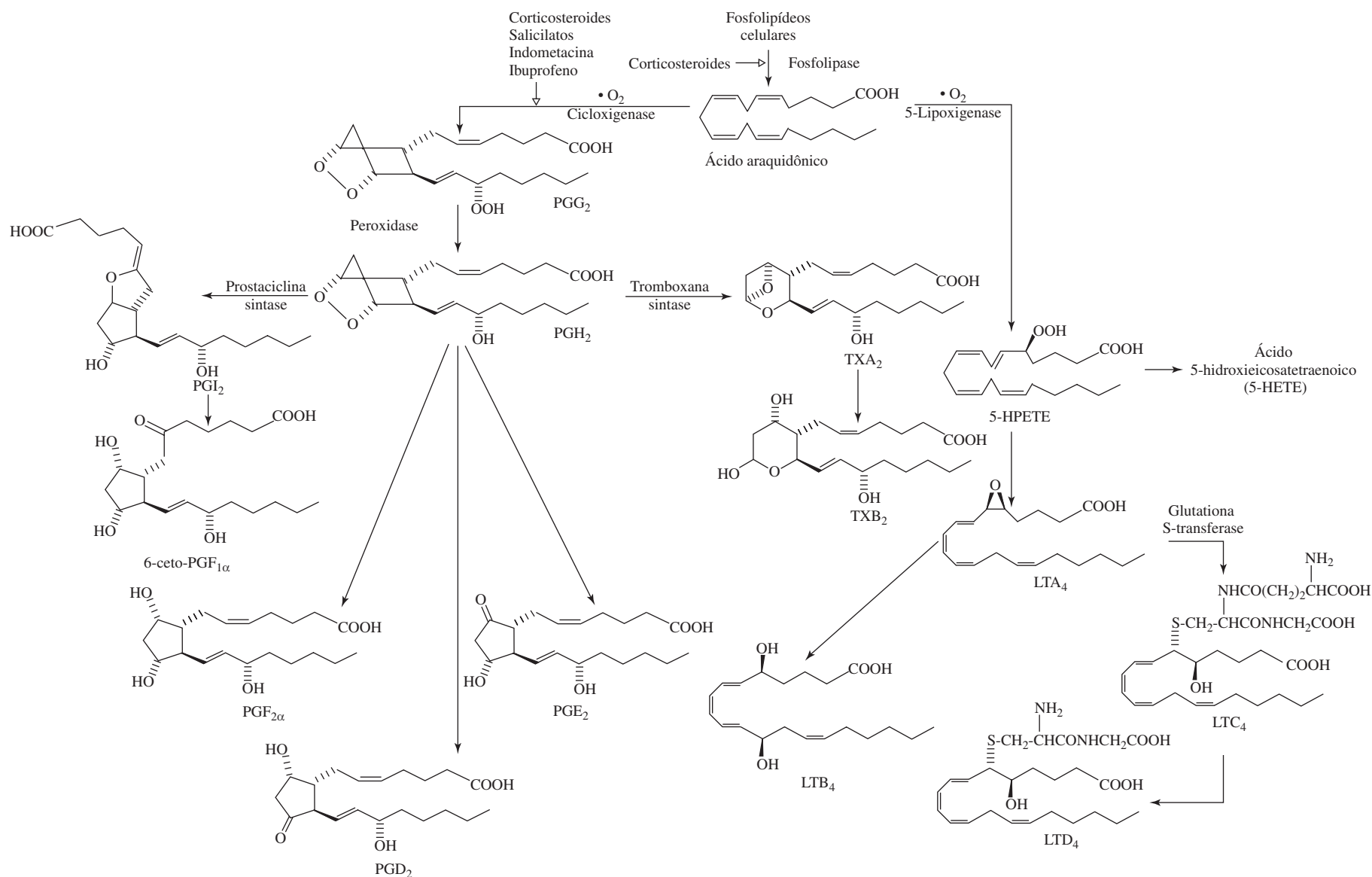
FIGURA 21-2 Vias de metabolismo do ácido araquidônico gerando prostaglandinas (PGs) e compostos correlatos, e leucotrienos (LTs). A via da ciclooxigenase leva à formação dos endoperóxidos cíclicos \text{PGG}_2 e \text{PGH}_2 e, subsequentemente, de prostaciclina ( \text{PGI}_2 ), tromboxana ( \text{TX} ) ou das PGs estáveis ( \text{E}_2 , \text{F}_{2\alpha} e \text{D}_2 ). A via da lipoxigenase resulta na formação de ácido 5-hidroperoxieicosatetraenoico (5-HPETE) e, subsequentemente, dos leucotrienos \text{A}_4 , \text{B}_4 , \text{C}_4 e \text{D}_4 . As setas com cabeças vazias (na parte superior do esquema) indicam as etapas metabólicas que são inibidas por corticosteroides ou anti-inflamatórios não esteroidais, como aspirina e ibuprofeno. Não foram incluídos o \text{LTE}_4 e o \text{LTF}_4 , nem outras vias de lipoxigenase.
