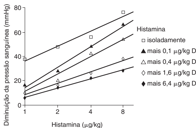
FIGURA 22-3 Curvas log dose-resposta ilustrando o antagonismo competitivo da histamina pela difenidramina (D). As diminuições da pressão arterial ( ordenadas ) causadas por doses intravenosas crescentes de histamina ( abscissas ) foram determinadas em cães anestesiados. Os animais receberam difenidramina (0,1 a 6,4 μg/kg) acompanhada pelas mesmas doses crescentes de histamina. (Dados de Chen G, Russel D: A quantitative study of blood pressure response to cardiovascular drugs and their antagonists. J Pharmacol Exp Ther 99:401-408, 1950.)
