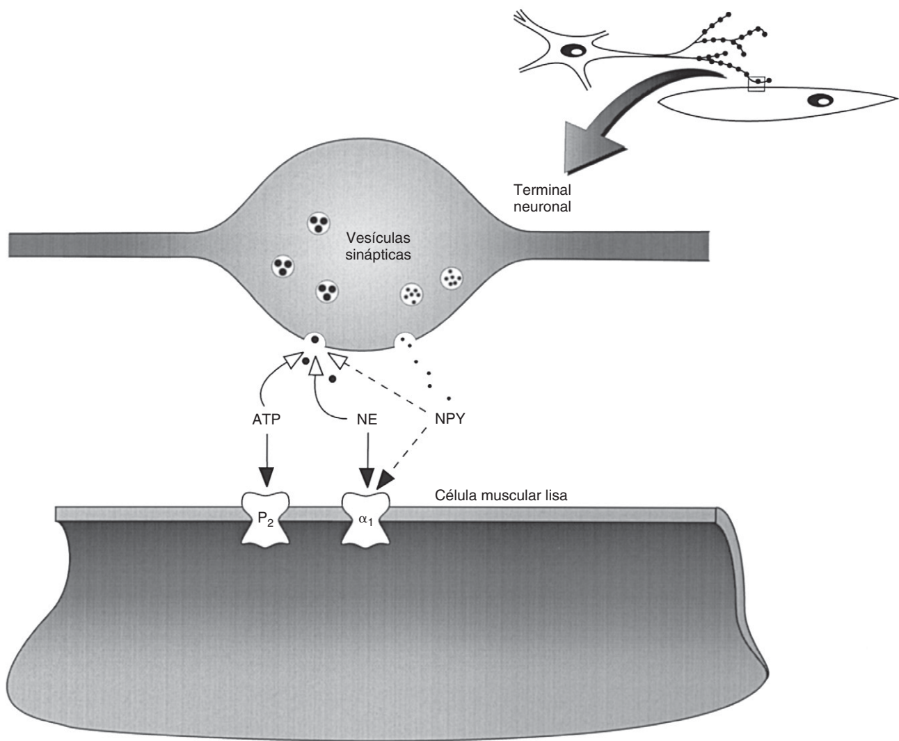
FIGURA 5-8 Coliberação de neurotransmissores e neuromoduladores. A norepinefrina (NE) e o ATP, armazenados nas mesmas vesículas, são liberados juntos a partir da varicosidade do neurônio simpático e estimulam ( setas cheias ) seus respectivos receptores, \alpha_1 e P_2 , na musculatura lisa. O neuropeptídeo Y (NPY), armazenado em vesículas independentes, também é liberado durante a estimulação do nervo simpático. Nessa situação, o NPY atua como neuromodulador ( setas tracejadas ), aumentando a atividade da NE. Os três agentes inibem liberação de NE adicional ( pontas de setas vazias ) por meio de efeito sobre receptores pré-juncionais (não representados).
