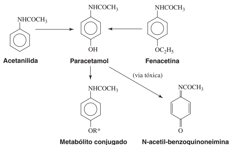
FIGURA 21-15 Estruturas e principais vias metabólicas do paracetamol, fenacetina e acetanilida. R*, Conjugados glicurônico (maior) e sulfato (menor). A N-acetil-benzoquinoneimina, produzida em grandes quantidades na superdosagem de paracetamol, forma um conjugado com a glutatona que acarreta depleção desta última.
