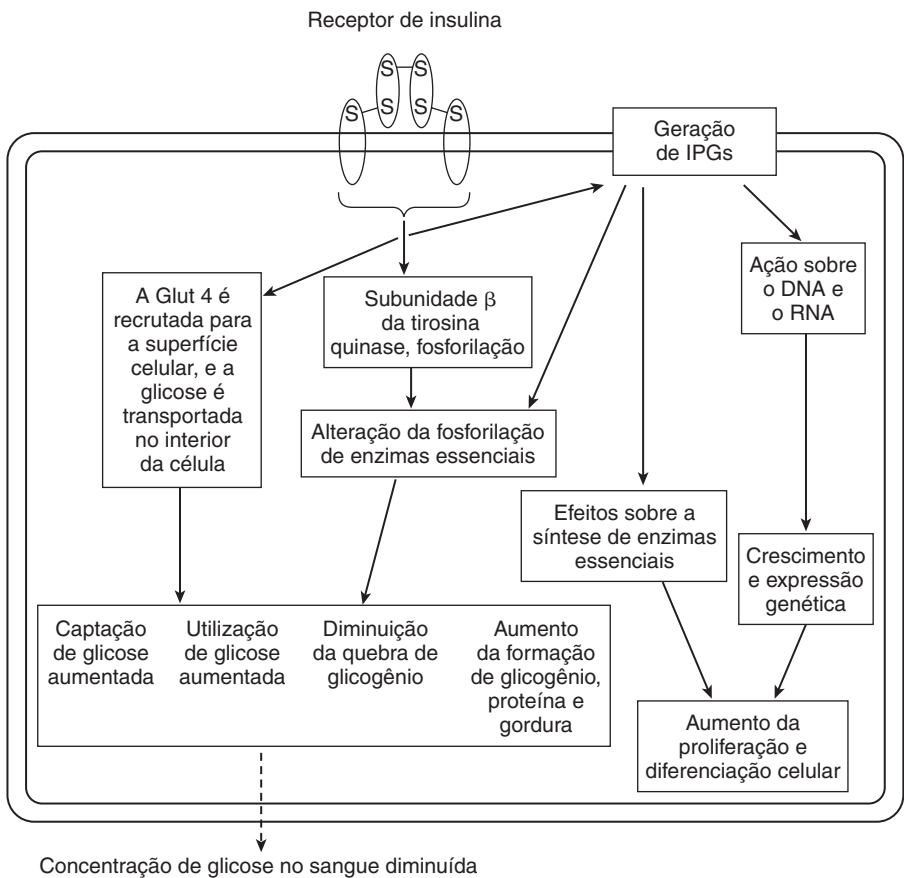
FIGURA 36-2 Vias de sinalização da insulina. Glut 4 , transportador de glicose 4.
