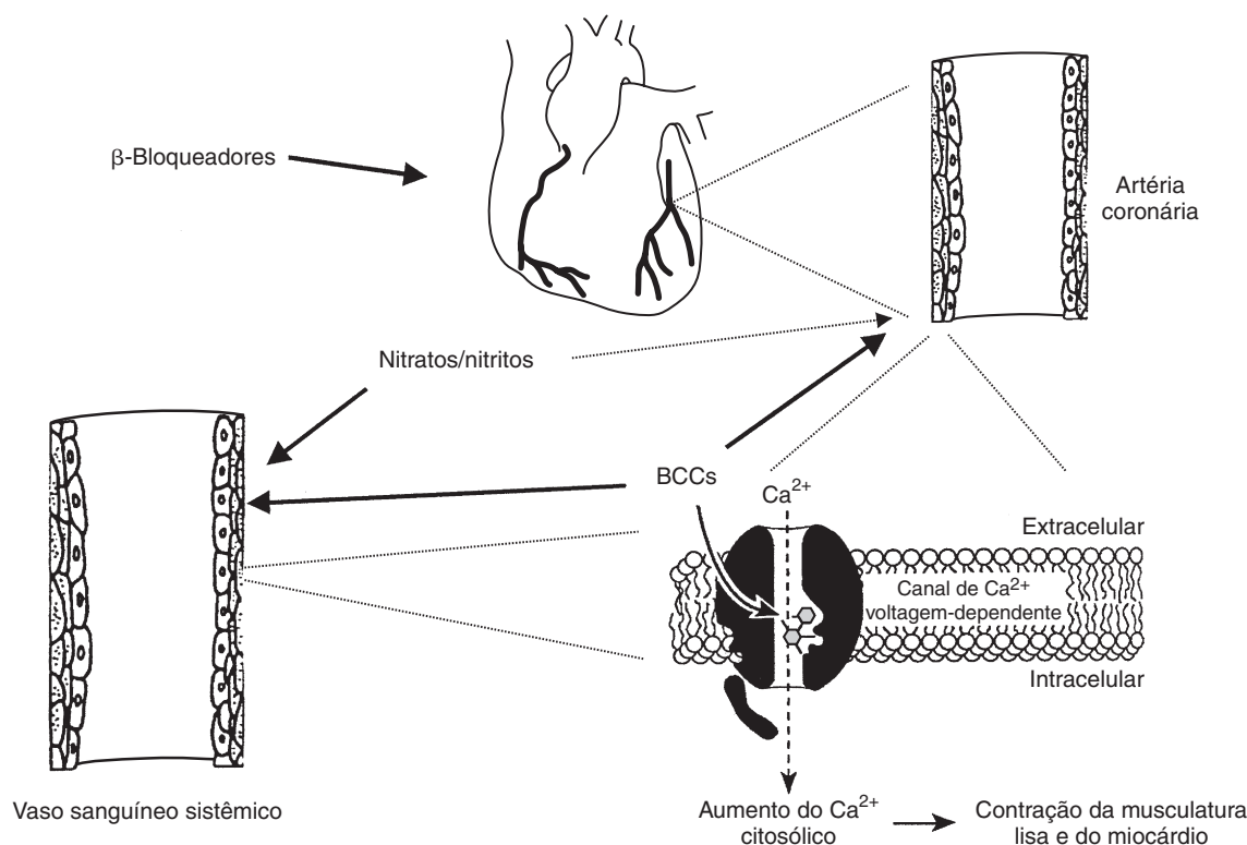
FIGURA 26-2 Sítios de ação para bloqueadores de receptores β-adrenérgicos, bloqueadores de canais de \text{Ca}^{2+} (BCCs) e nitratos/nitritos. Os β-bloqueadores reduzem a frequência e a contratilidade cardíaca, reduzindo a demanda energética e de oxigênio do coração. Os BCCs reduzem a vasoconstrição em vasos coronarianos e não coronarianos, aumentando o fluxo sanguíneo pelas coronárias e reduzindo a carga cardíaca. Os nitratos/nitritos agem principalmente sobre vasos sanguíneos sistêmicos, reduzindo a carga cardíaca. Seu efeito sobre as artérias coronárias é de importância menor no alívio da angina clássica, mas tem desempenho importante na angina variante. Três níveis anatômicos estão ilustrados: anatomia cardíaca, camadas celulares das paredes dos vasos sanguíneos e a membrana celular da musculatura lisa de um vaso sanguíneo mostrando um canal de \text{Ca}^{2+} e o efeito dos BCCs na inibição da entrada de \text{Ca}^{2+} .
