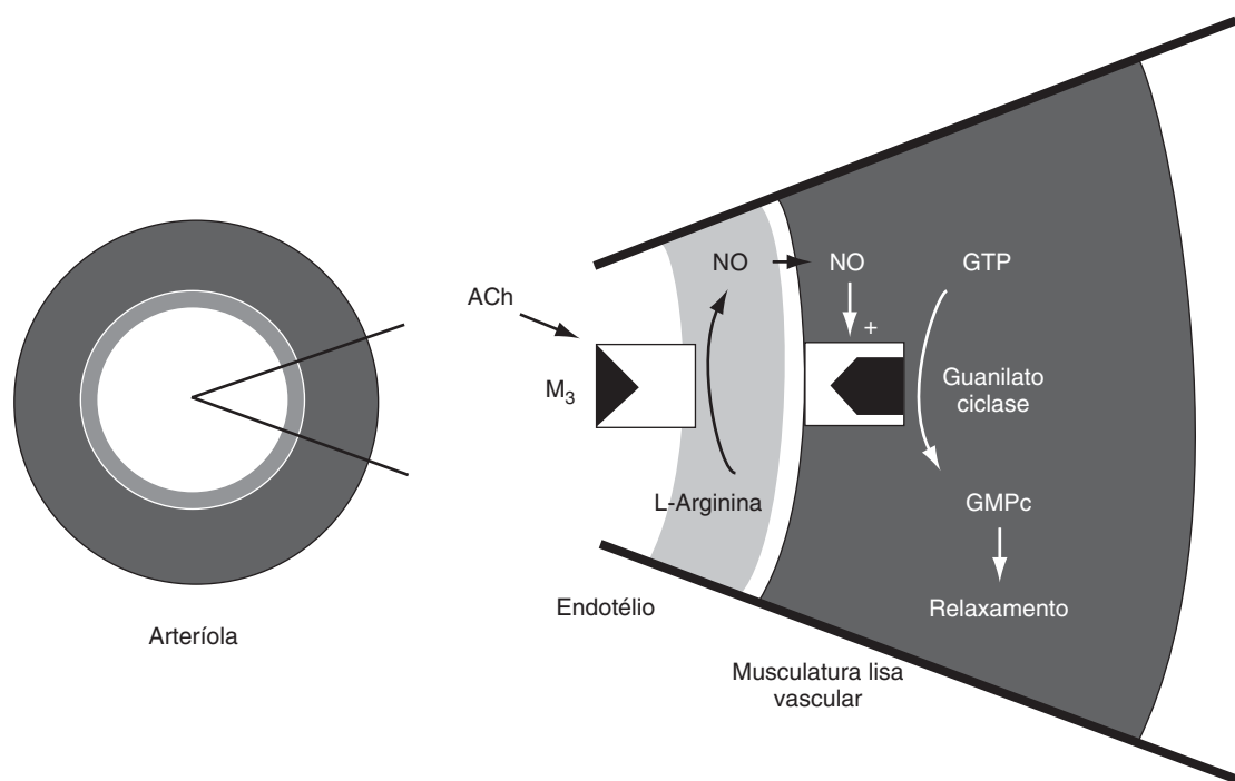
FIGURA 8-3 Mecanismos de relaxamento vascular por agonistas de receptores muscarínicos. O agente muscarínico acetilcolina (ACh) liga-se ao seu receptor ( M_3 ) no endotélio vascular íntimo. O óxido nítrico (NO) recém-sintetizado difunde-se para a musculatura lisa vascular, onde estimula a formação de guanosina 3',5'-monofosfato cíclico (GMPc) a partir de guanosina trifosfato (GTP).
